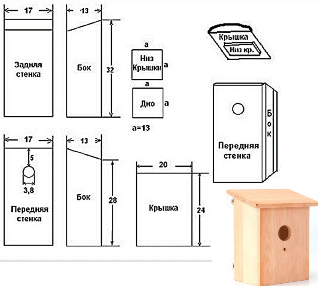
Чертеж 1. «Скворечник с односкатной крышей»
